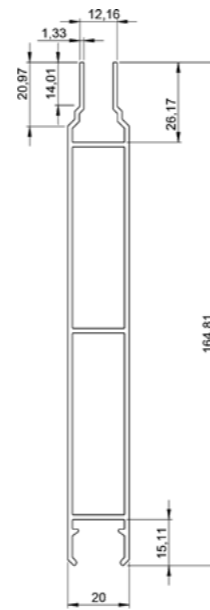
Panel Profil Kesiti
