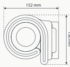
Duvar Montaj
